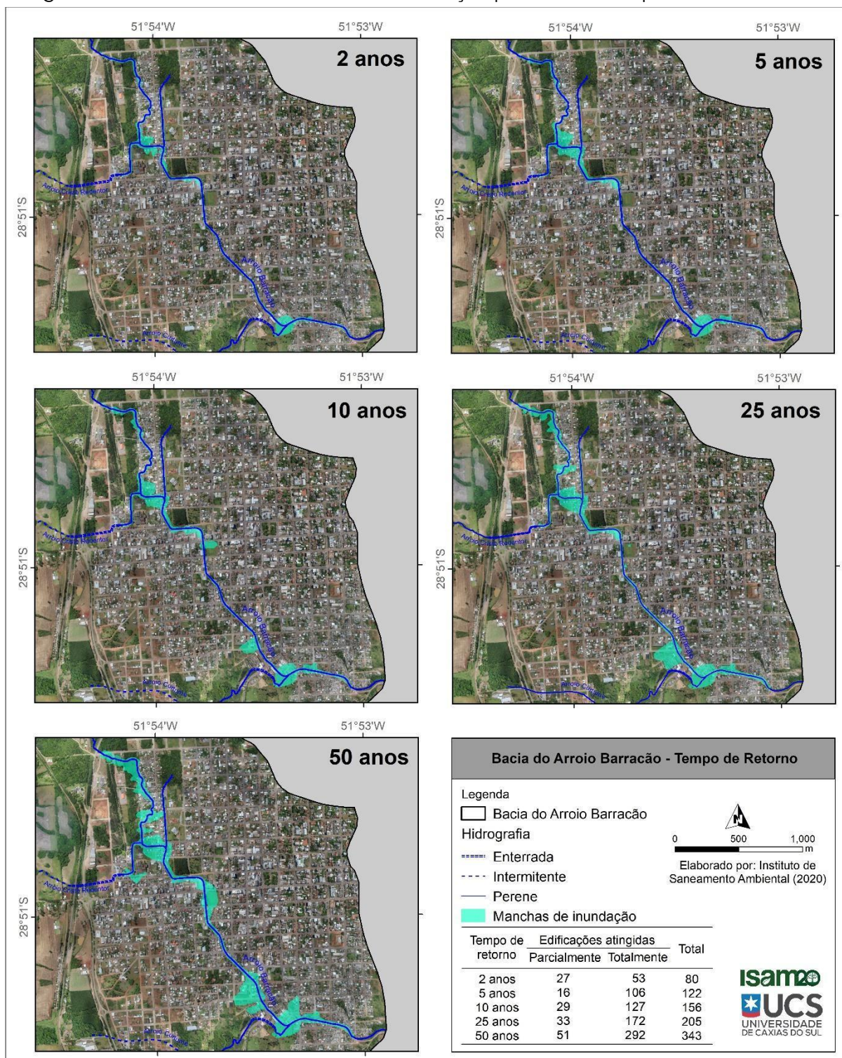
Figura 92 – Resultado das manchas de inundação para diferentes períodos de retorno
