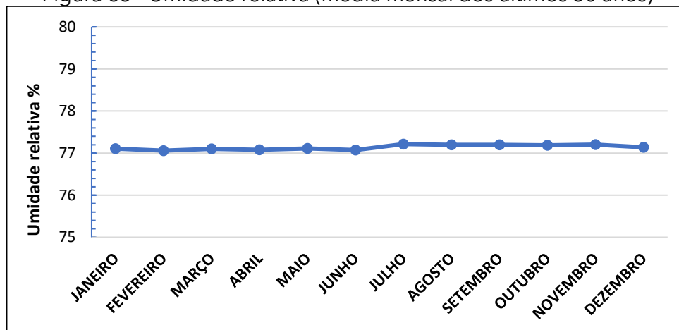
Figura 65 - Umidade relativa (média mensal dos últimos 30 anos)
