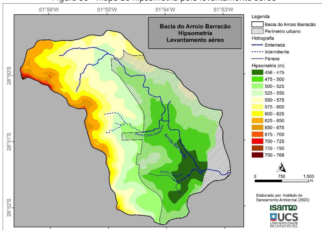
Figura 36 - Mapa de hipsometria pelo levantamento aéreo
