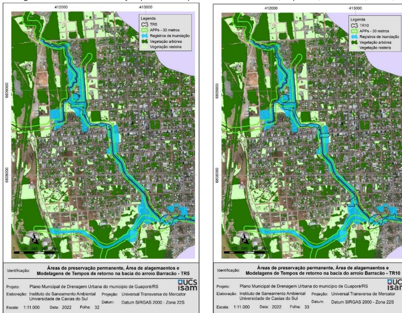
Figura 96 - Área de inundação para os tempos de retorno 5 anos (esquerda) e 10 anos (direita)
