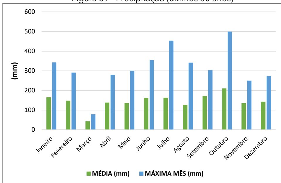
Figura 69 - Precipitação (últimos 30 anos)
