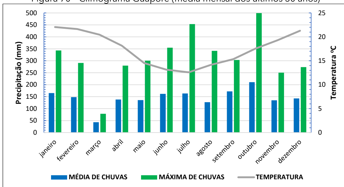
Figura 70 – Climograma Guaporé (média mensal dos últimos 30 anos)
