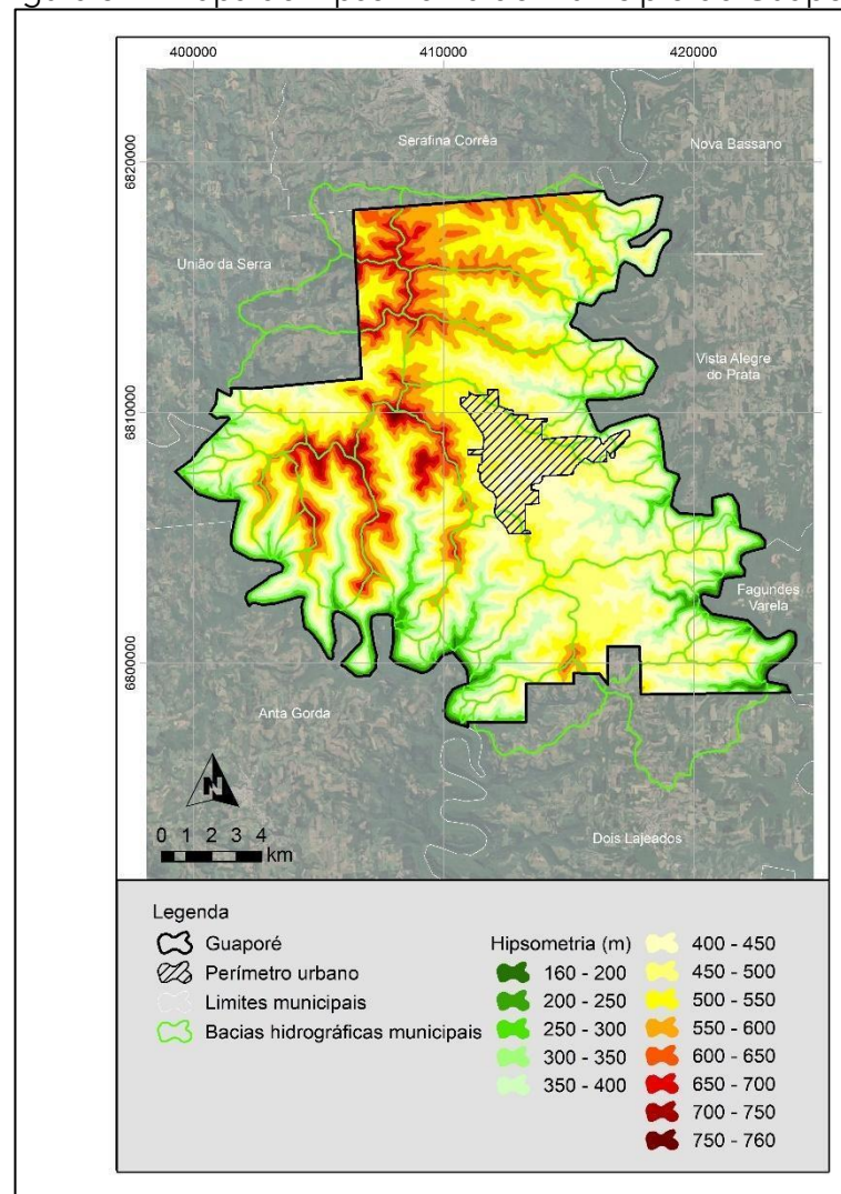
Figura 34 – Mapa de hipsometria do município de Guaporé
