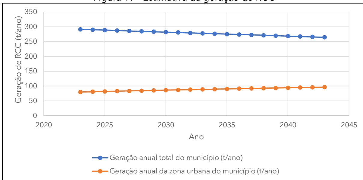
Figura 19 - Estimativa da geração de RCC
