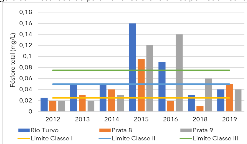
Figura 63 – Resultado do parâmetro fósforo total nos pontos amostrados
